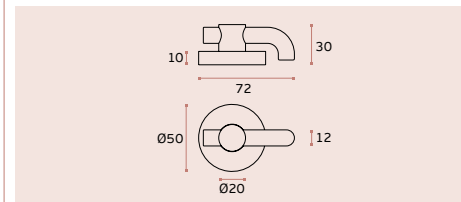
SM.030 Fecho para wc com indicador "livre-ocupado" / Bathroom latch for sliding door with indicator / Cierre de baño para puertas correderas con indicador. EN 1.4301 Satinado / Satin / Satin
