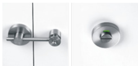
SM.026 Fecho com indicador "livre-ocupado" / Bathroom latch with indicator / Cierre de baño con indicador. EN 1.4301 Satinado / Satin / Satin
