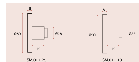
SM.011.25 SM.011.19 Suporte de tubo com fixação à parede / Wall mounting tube support / Soporte de tubo con sujeción a pared. EN 1.4301 Satinado / Satin / Satin
