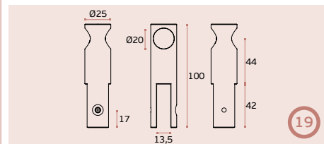
SM.022 Suporte superior para painel / Upper panel holder / Soporte superior para panel. EN 1.4301 Satinado / Satin / Satin
