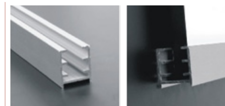
SM.103 Perfil para painel de 13mm / Profile for 13mm panel / Perfil para panel de 13mm. Alumínio / Aluminium / Aluminio Cor natural / Natural color / Color natural
