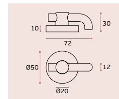
SM.029 Fecho com indicador "livre-ocupado" / Bathroom latch with indicator / Cierre de baño con indicador. EN 1.4301 Satinado / Satin / Satin
