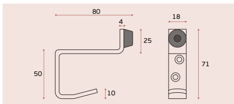
IN.14.529 Cabide duplo com batente de porta / Double hook with door stopper / Colgador doble con tope de puerta. EN 1.4301 Satinado / Satin / Satin
