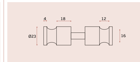
SM.020 Puxador de porta duplo, anti-vandalismo / Back to back door knob, anti vandalism fixing / Tirador de puerta doble, anti vandalismo. EN 1.4372 Satinado / Satin / Satin
