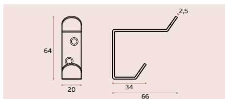
IN.14.530.ECO Cabide duplo / Double hook / Colgador doble. EN 1.4372 Satinado / Satin / Satin
