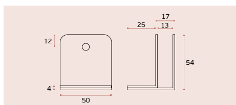
SM.014 Suporte para painel / Panel holder / Soporte para panel. EN 1.4301 Satinado / Satin / Satin
