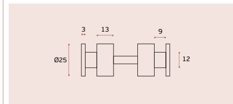
SM.019 Puxador de porta duplo, anti-vandalismo / Back to back door knob, anti vandalism fixing / Tirador de puerta doble, anti vandalismo. EN 1.4301 Satinado / Satin / Satin
