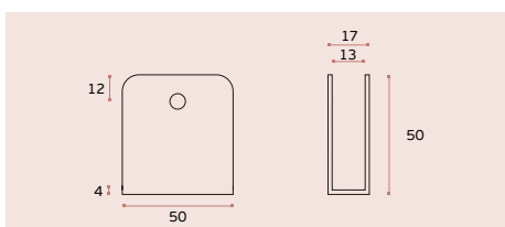
SM.024 Suporte para painel / Panel holder / Soporte para panel. EN 1.4301 Satinado / Satin / Satin
