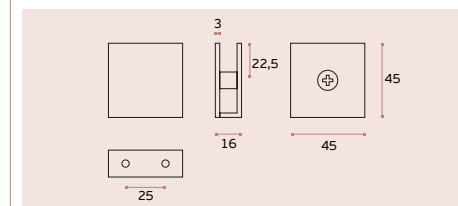
SM.039 Suporte para painel / Panel holder / Soporte para panel. EN 1.4301 Satinado / Satin / Satin
