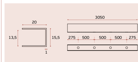
SM.101 Perfil em "U" para painel de 13mm / "U" shape profile for 13mm panel / Perfil en "U" para panel de 13mm. EN 1.4301 Satinado / Satin / Satin
