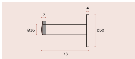
SM.008 Cabide / batente de porta anti-vandalismo / Hook / door stopper concealed fixing / Percha / tope de puerta anti-vandalismo. EN 1.4301 Satinado / Satin / Satin
