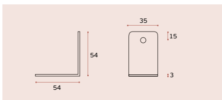
SM.044 Suporte para painel / Panel holder / Soporte para panel. EN 1.4301 Satinado / Satin / Satin
