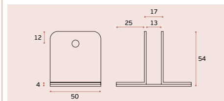
SM.034 Suporte para painel / Panel holder / Soporte para panel. EN 1.4301 Satinado / Satin / Satin
