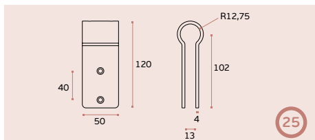
SM.002 Suporte superior para painel / Upper panel holder / Soporte superior para panel. EN 1.4301 Satinado / Satin / Satin
