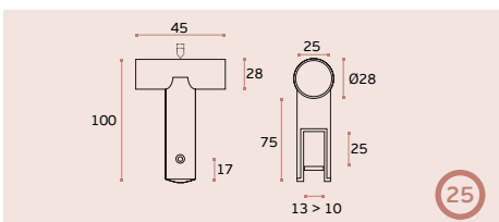
SM.012.90 SM.012.180 Suporte superior para painel / Upper panel holder / Soporte superior para panel. EN 1.4301 Satinado / Satin / Satin
