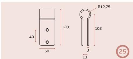
SM.002.ECO Suporte superior para painel / Upper panel holder / Soporte superior para panel. EN 1.4372 Satinado / Satin / Satin
