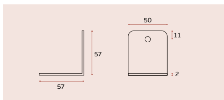
SM.004 Suporte para painel / Panel holder / Soporte para panel. EN 1.4301 Satinado / Satin / Satin
