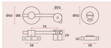
SM.027 Fecho para wc com indicador "livre-ocupado" para portas de correr / Bathroom latch for sliding door with indicator / Cierre de baño para puertas correderas con indicador. EN 1.4301 Satinado / Satin / Satin
