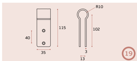
SM.002.19 Suporte superior para painel / Upper panel holder / Soporte superior para panel. EN 1.4301 Satinado / Satin / Satin
