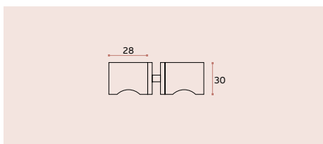
IN.75.030 Puxadores para portas de vidro ou fenólico / Knobs for glass or phenolic doors / Pomos para puerta de cristal o fenolico. Material EN 1.4301 Satinado / Satin / Satin
