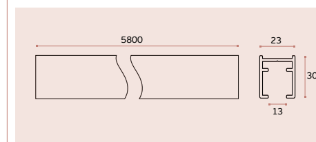
SM.103 Perfil para painel de 13mm / Profile for 13mm panel / Perfil para panel de 13mm. Alumínio / Aluminium / Aluminio Cor natural / Natural color / Color natural
