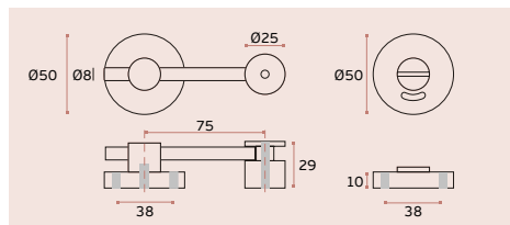
SM.026 Fecho com indicador "livre-ocupado" / Bathroom latch with indicator / Cierre de baño con indicador. EN 1.4301 Satinado / Satin / Satin
