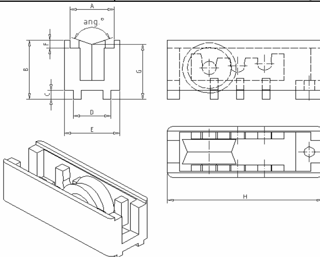
COTAS (mm)
