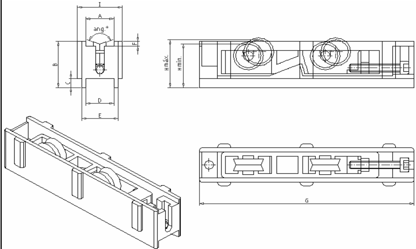
COTAS (mm)
